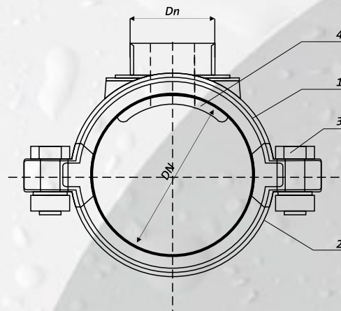
Обойма NOBW с внешней резьбой
