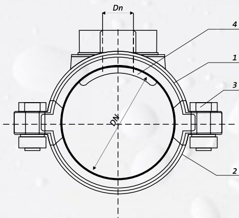
Обойма NOBW с внутренней резьбой
